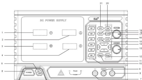
前面板图
